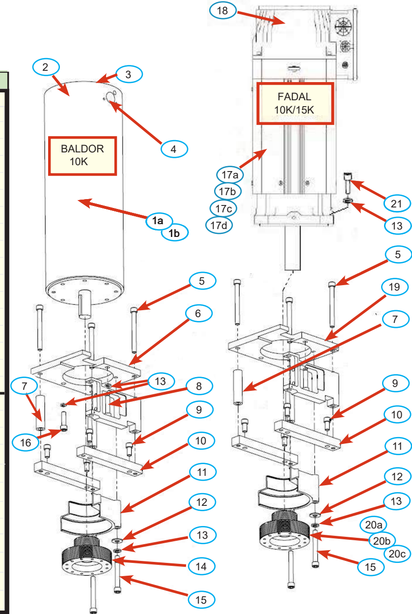
SPINDLE MOTOR
