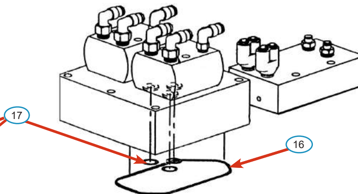
HYDRAULIC ACTUATORS
