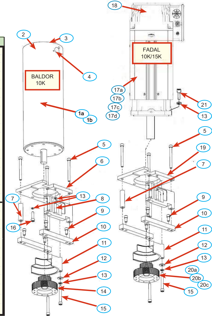
SPINDLE MOTOR
