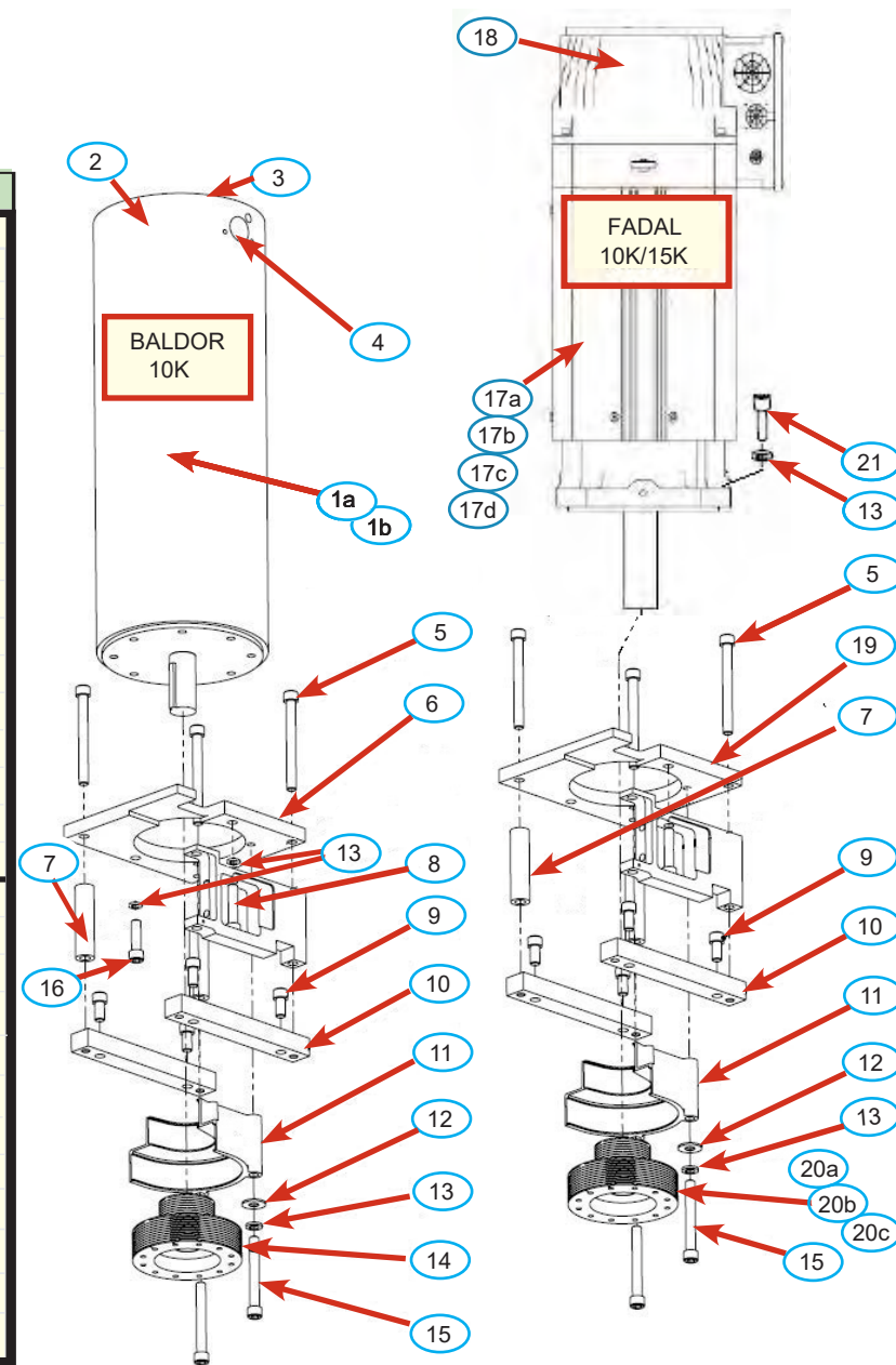
SPINDLE MOTOR
