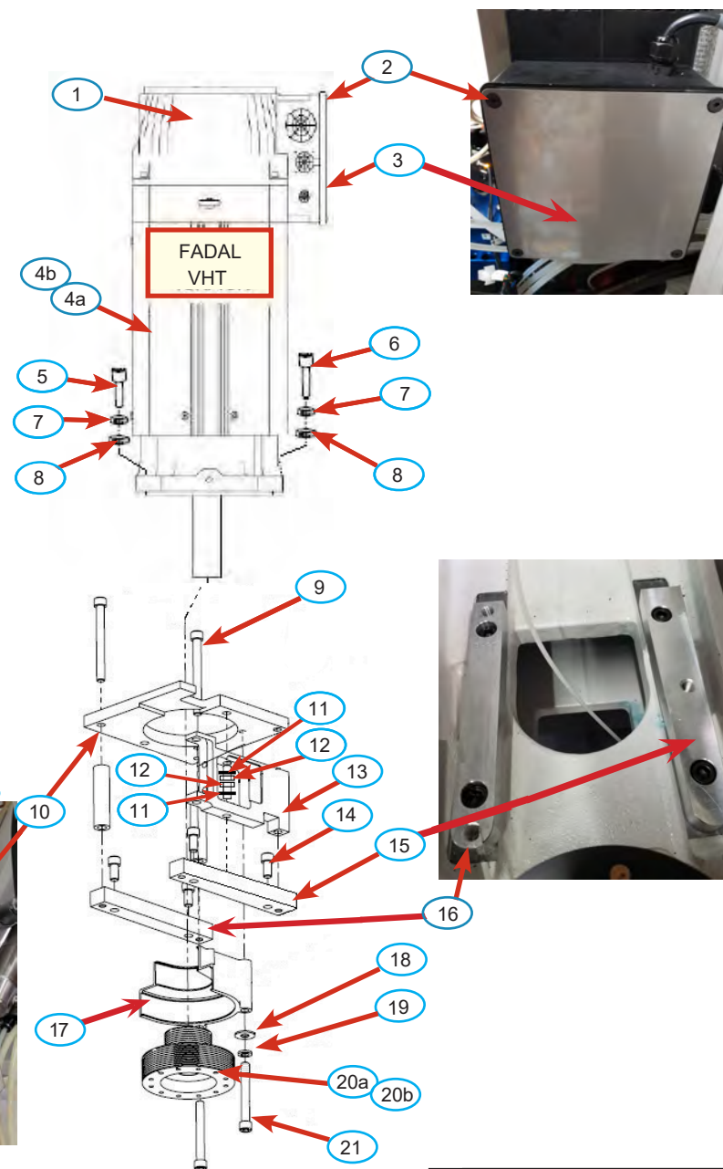
VHT SPINDLE MOTOR
