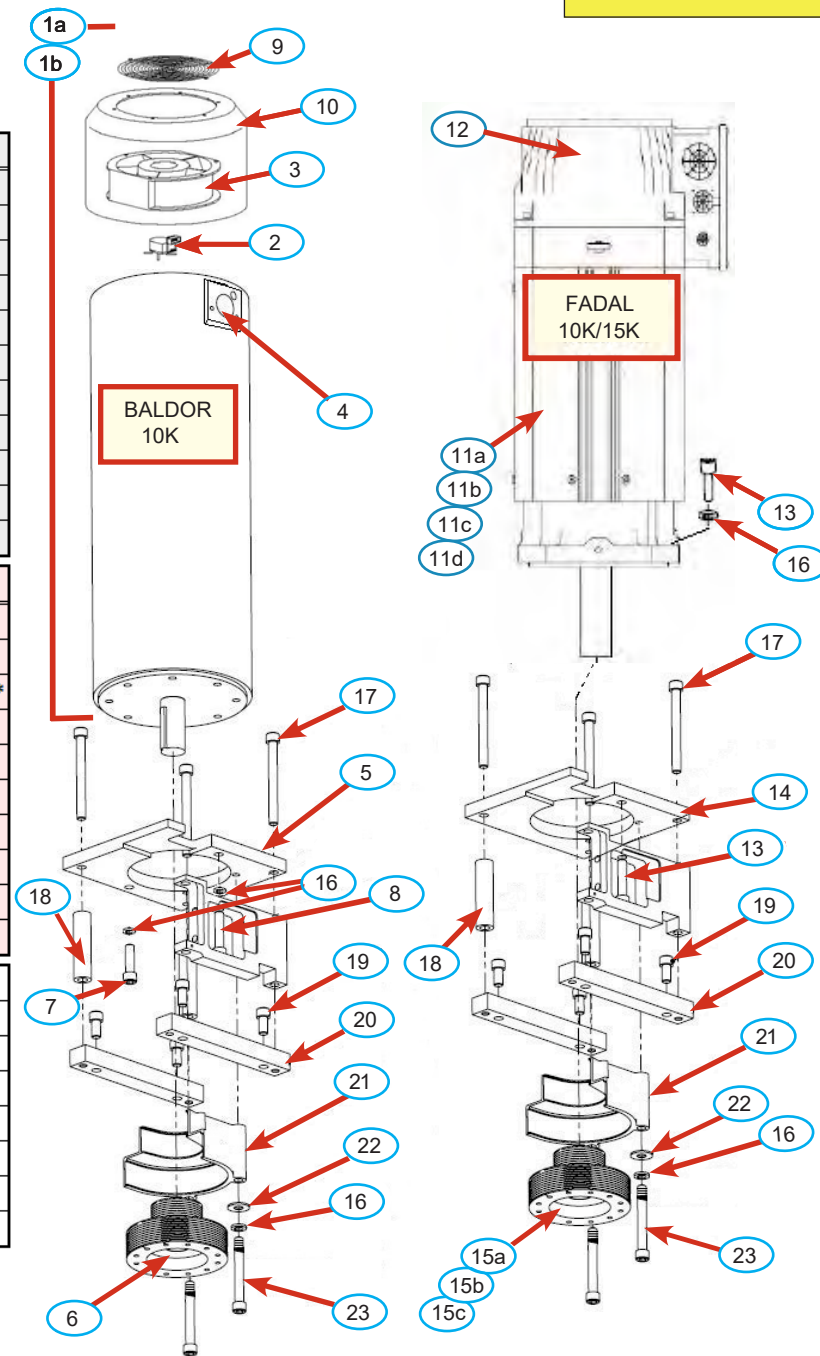
SPINDLE MOTOR
