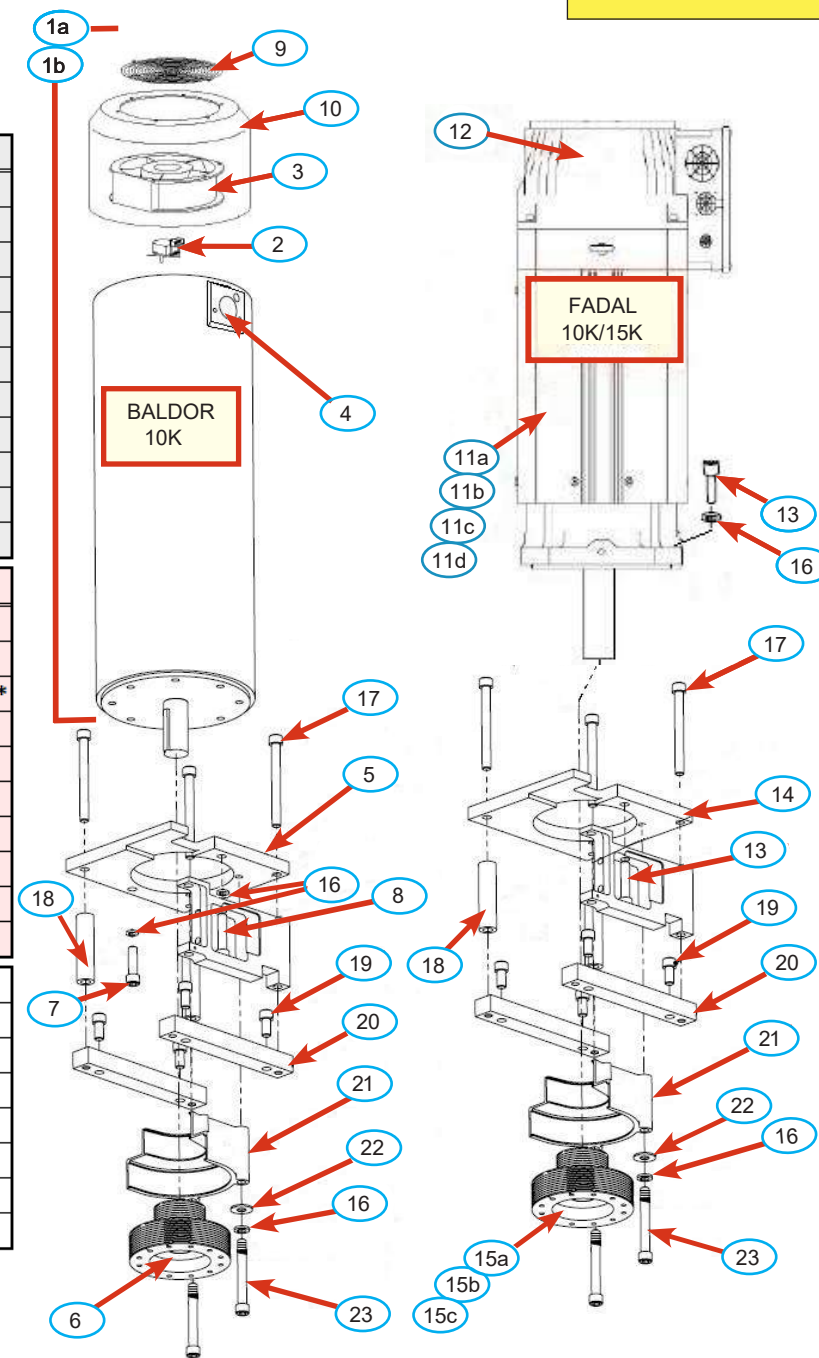
SPINDLE MOTOR
